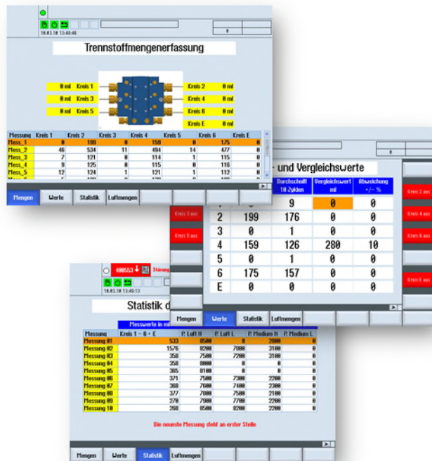
imagen: supervisión de la capacidad del flujo para 6 circuitos de lubricante integrado en sistemas de pulverización
