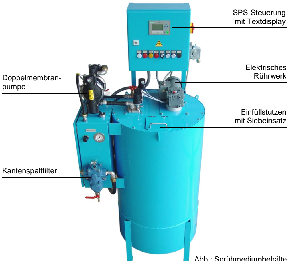
Abb.: Sprühmediumbehälter 200 Liter
